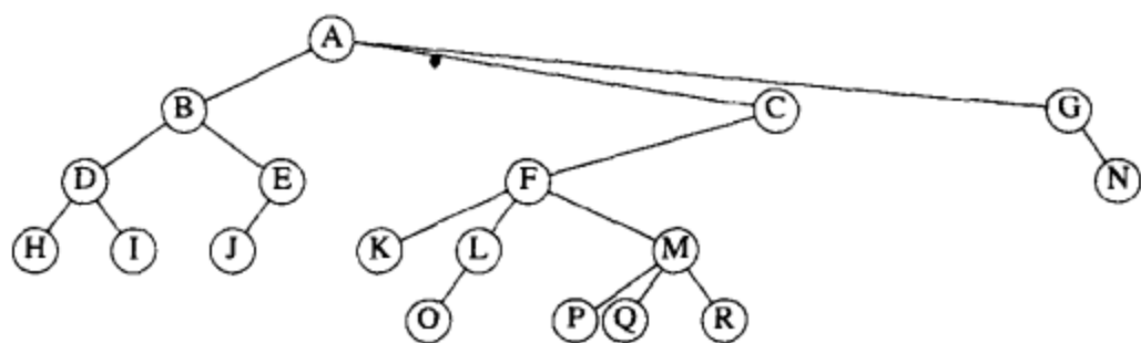
图 4-62 练习 4.39 中的树
