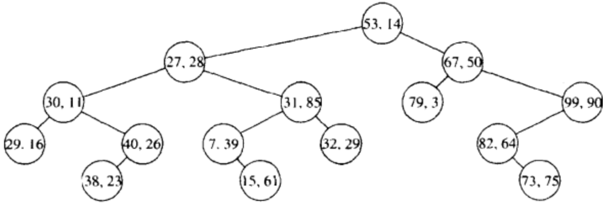
图 12-42 2-d 树示例
