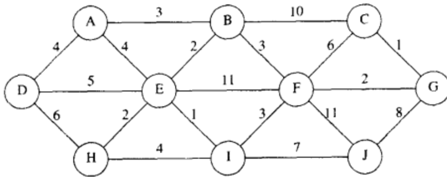
图 9-82
