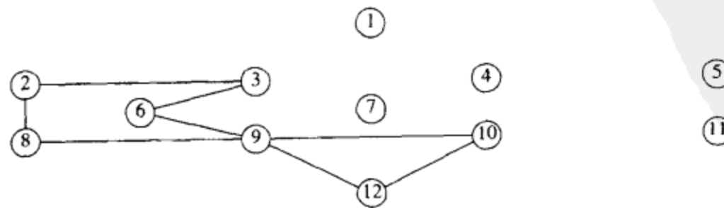
图 9-72 遍历 5, 4, 1, 3, 7, 4, 11, 10, 7, 9, 3, 4, 10, 5 后的图
