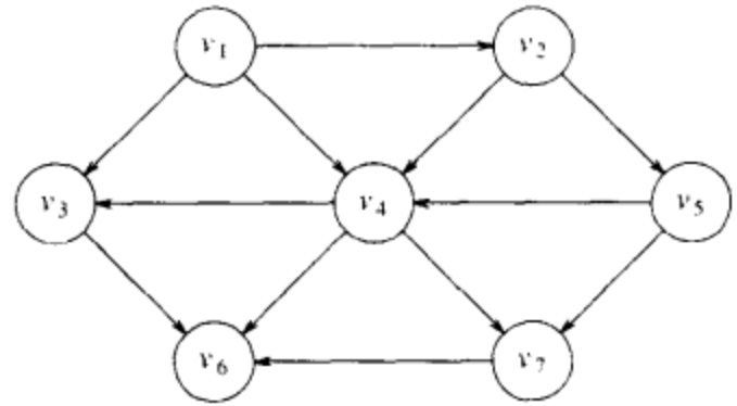
图 9-4 一个无圈图
