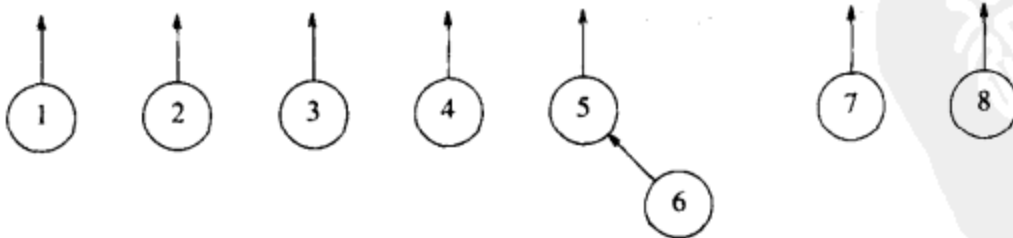
图 8-2 在 Union(5, 6) 之后
