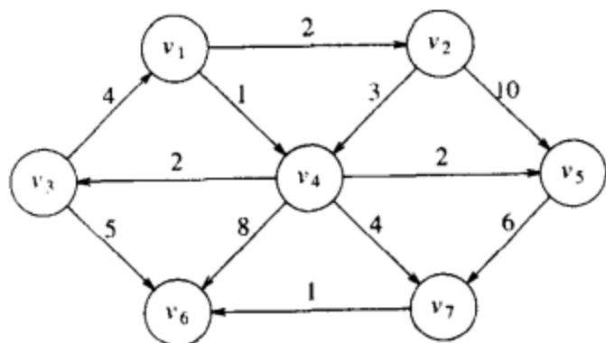
图 9-20 有向图 G
