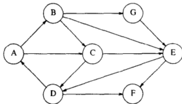
图 9-84
