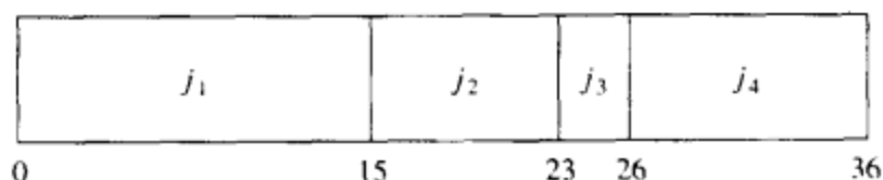
图 10-2 1号调度
