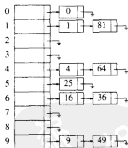
图 5-6 分离链接散列表
