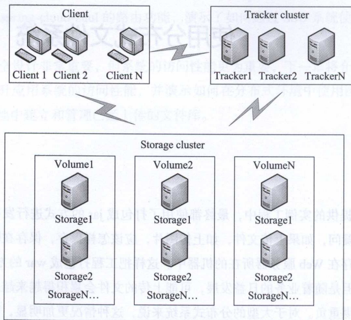
图 7-1 FastDFS 服务器网络拓扑
