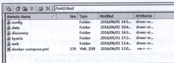
图 9-1 发布服务的目录结构
