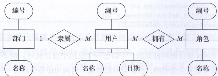
图 4-4 实体 - 关系模型设计
